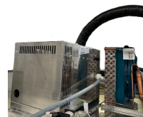
Hocheffizienter Dampfkessel (Dampferzeugung von 2-2,6 kg/h)
