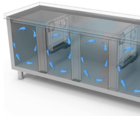
Circolazione dell'aria in cella
